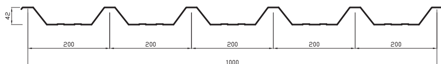
Chapa perfilada 42/200
